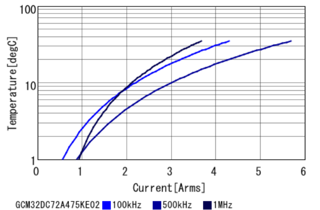
温度上升由于脉动电流特性
